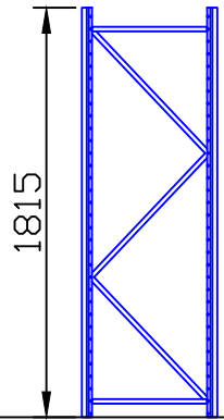
55立柱片安装图
