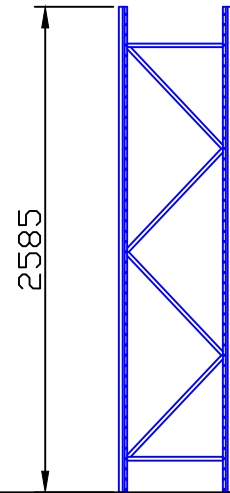
55立柱片安装图
