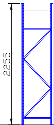
55立柱片安装图
