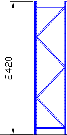
55立柱片安装图
