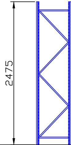
55立柱片安装图
