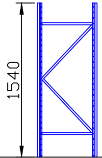
55立柱片安装图
