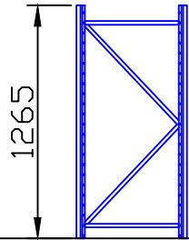
55立柱片安装图
