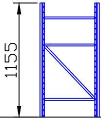
55立柱片安装图
