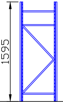
55立柱片安装图
