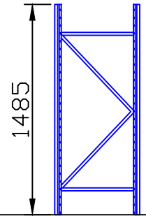
55立柱片安装图
