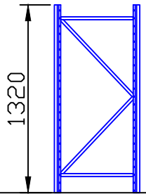
55立柱片安装图
