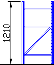
55立柱片安装图
