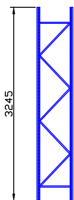
55立柱片安装图
