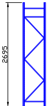
55立柱片安装图
