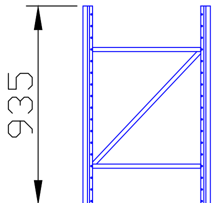
55立柱片安装图
