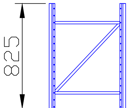
55立柱片安装图
