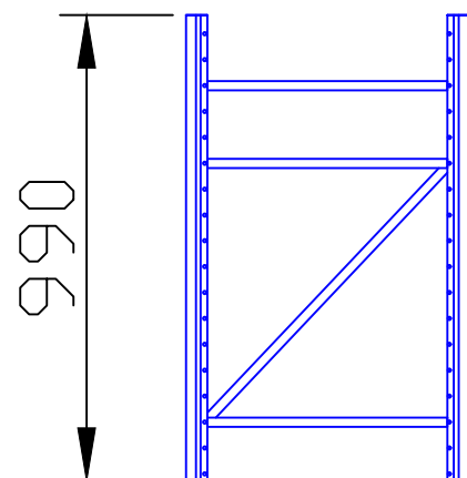
55立柱片安装图
